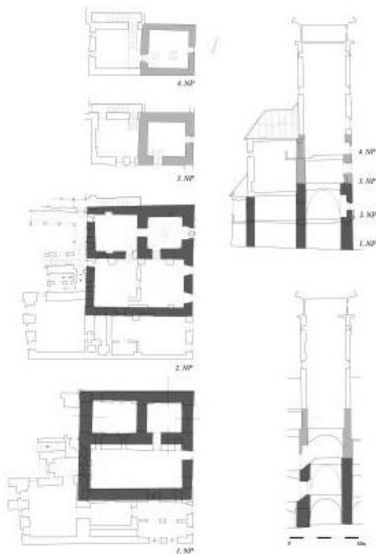
Obr. 6: Brno, Radnická 10 – „Stará radnice. Půdorys 1 NP, 2 NP, řezy věží. Tmavě šedá – rozsah nejstarší stavební fáze, světle šedá – předpokládaný rozsah nejstarší stavební fáze.
