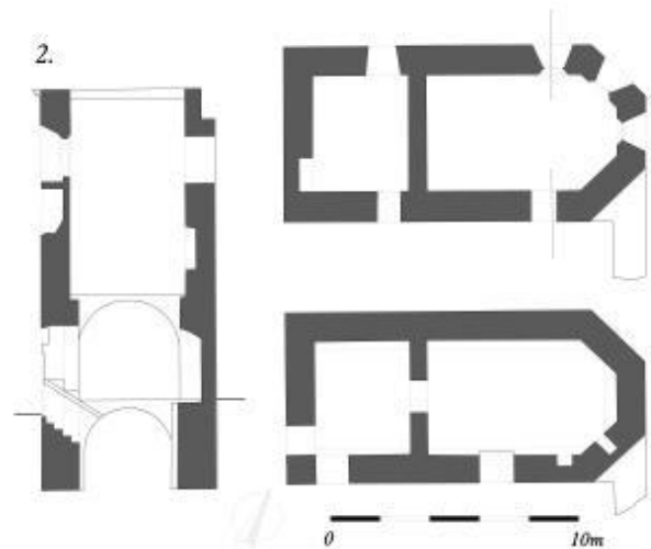
Obr. 4: Brno, Dominikánské náměstí. 1 – půdorys přízemí domu cisterciáček, Královské kaple a oratoře z r. 1791, a) oratoř; b) věž při domu cisterciáček; 2 – půdorys a řezy 1 NP a 2 NP oratoře – kaple sv. Prokopa (Archiv města Brna fond U9, Fa 20, Fa 21).
