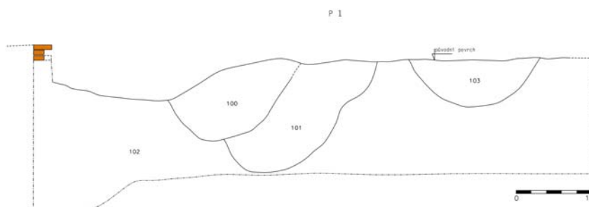
Obr. 3 – kresebná dokumentace řezu P1.
